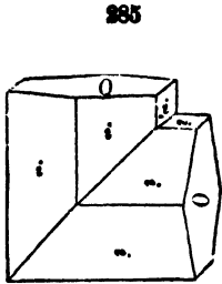
Calcite.
